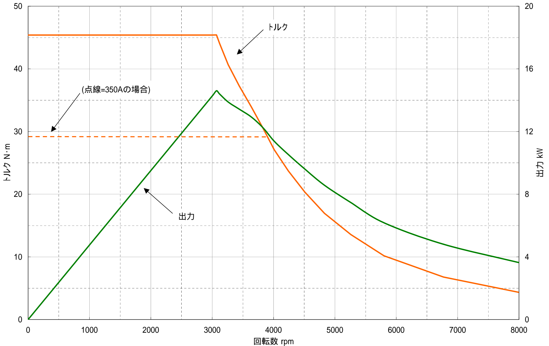
図 アドバンスドD.C. 140-01-4005 性能曲線 (DC48Volts - 500Amps)
