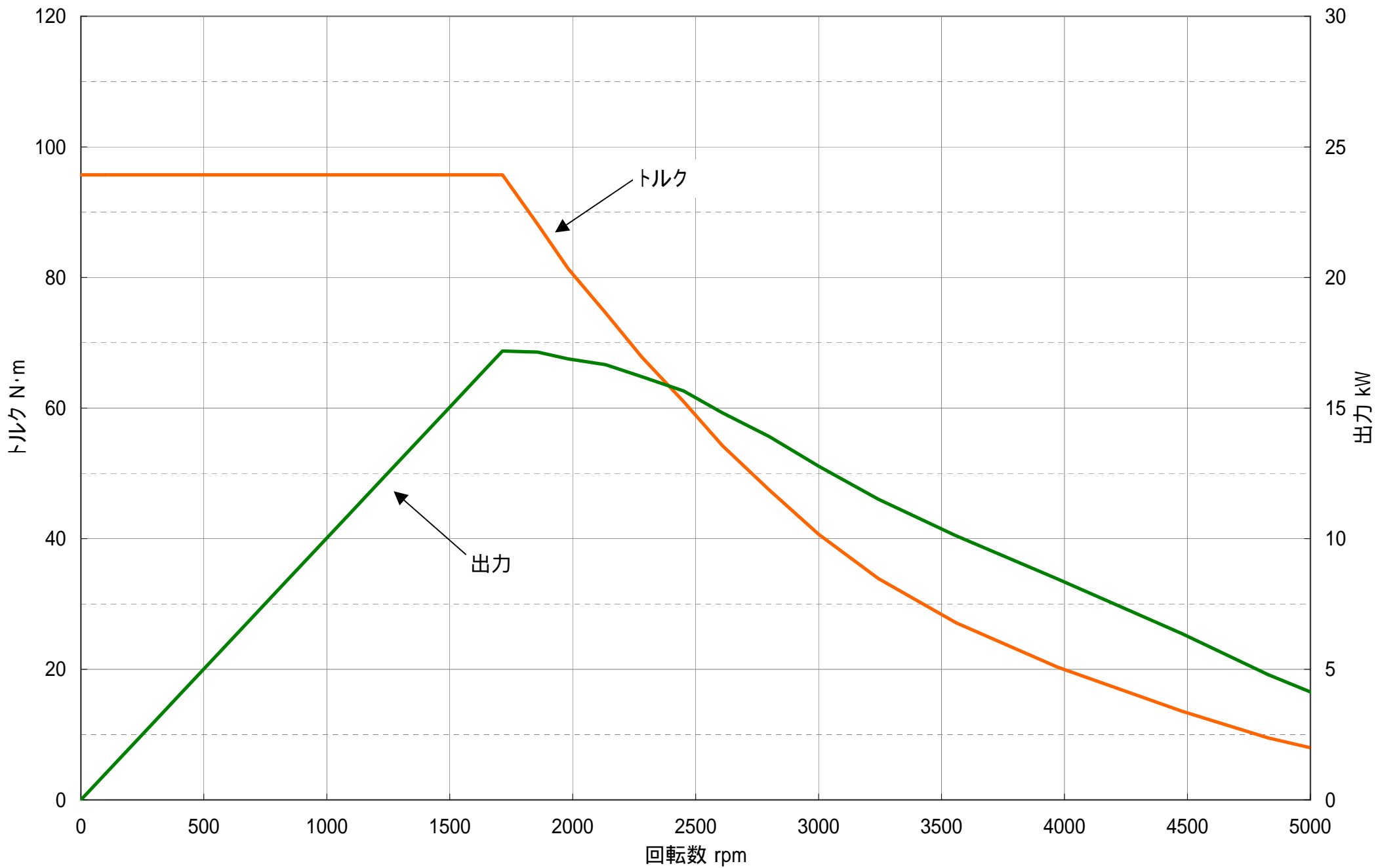
図 アドバンスD.C. A89-4001、A00-4009 性能曲線 (72Volts-500Amps)
